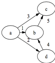
FIGURE: Expression de la matrice d'incidence précédente
