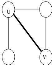
L'arête (u,v) n'est pas un pont
