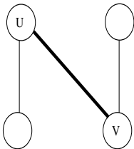
L'arête (u,v) est un pont
